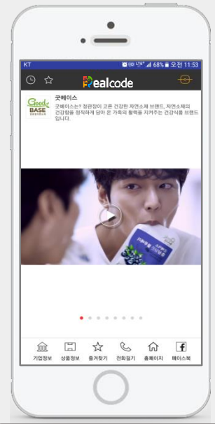
정품인증 완료화면(재생화면)
