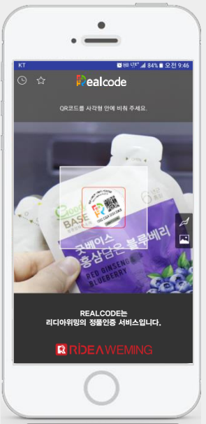
리얼코드 인식화면
